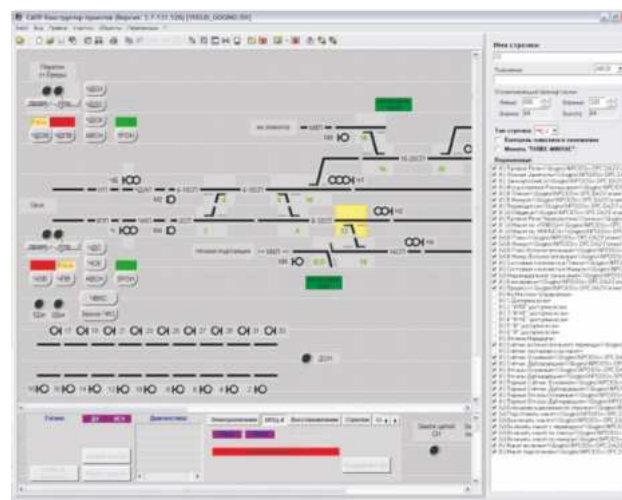
Адаптация ПО верхнего уровня МПЦ-И
