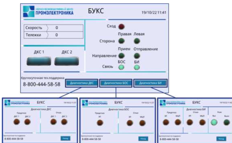
Интерфейс постового терминала БУКС
