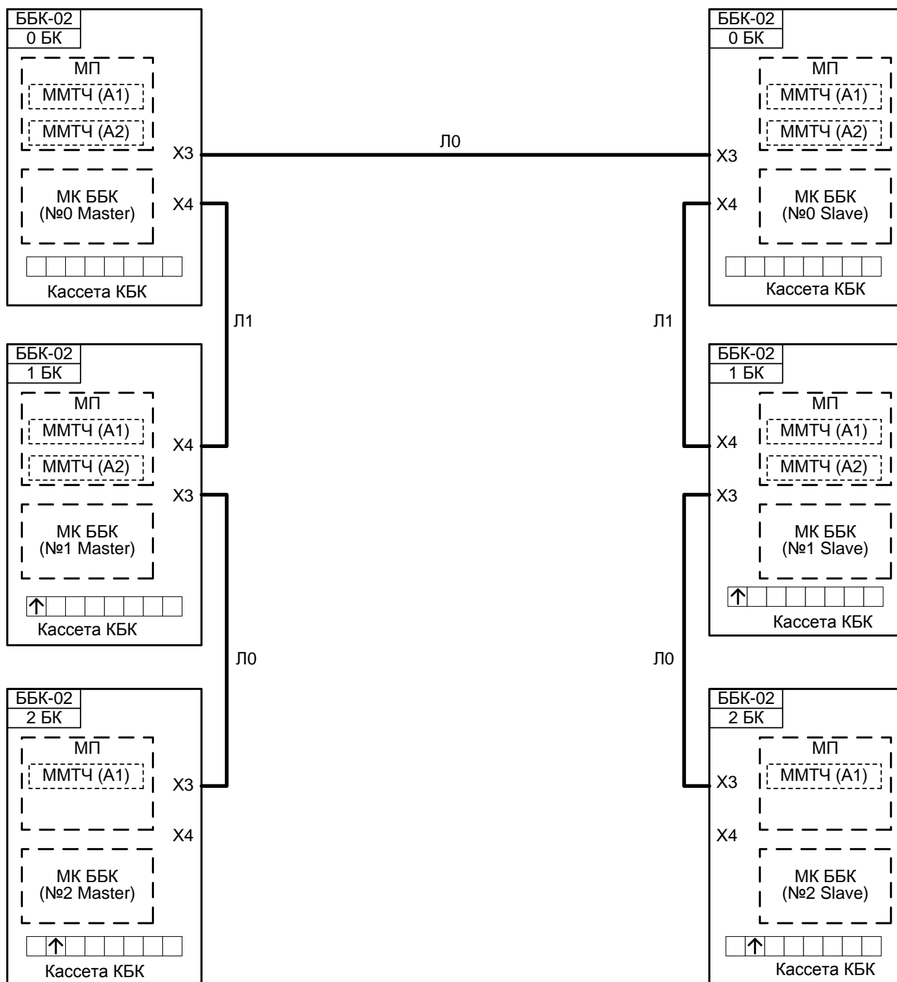
Рисунок Г.1 – Функциональная схема каскадного включения блоков БК-02 в общем канале связи
