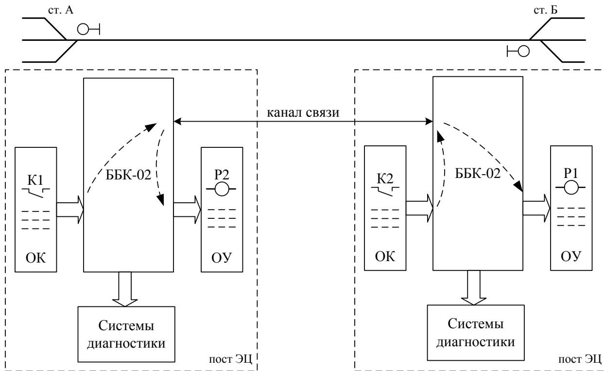
Рисунок 1 – Структура обмена данными между блоками БК-02
