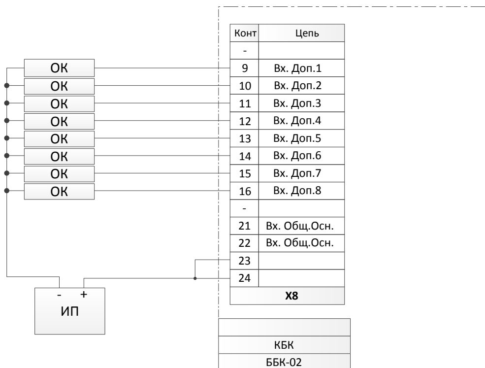
Рисунок 4 – Схема подключения к дополнительным входам блока ББК-02
