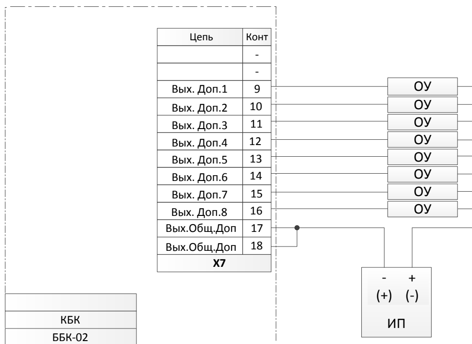
Рисунок 6 – Схема включения дополнительных выходов блока ББК-02
