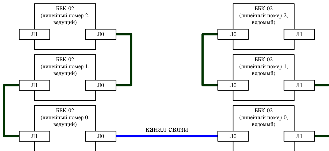
Рисунок 2 – Схема каскадного включения блоков БК-02
