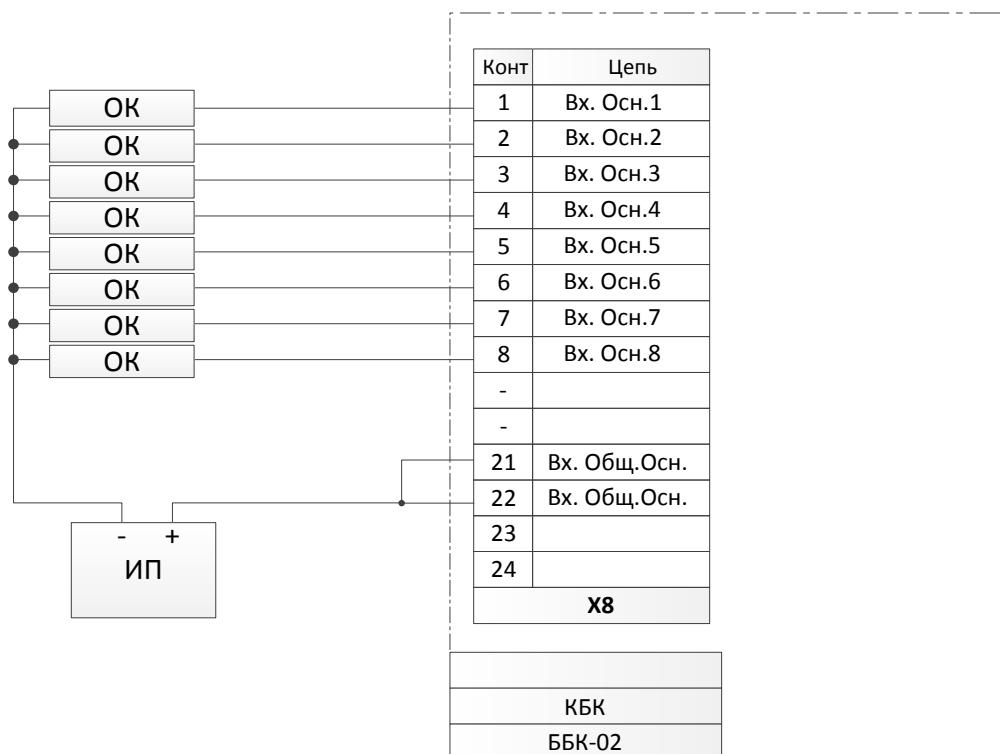
Рисунок 3 – Схема подключения к основным входам блока ББК-02
