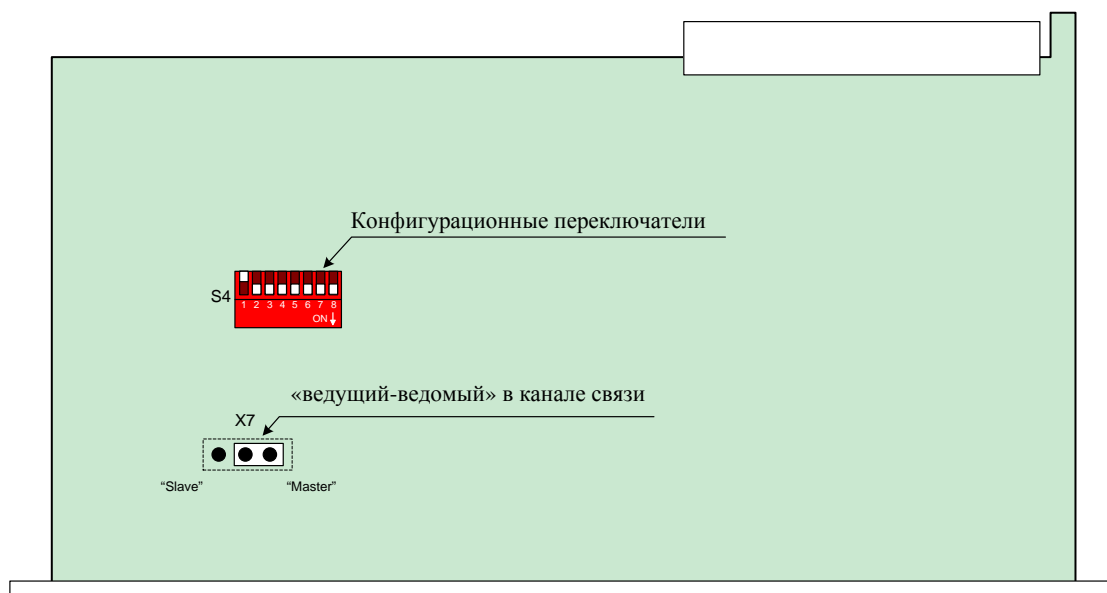
Рисунок 9 – Размещение органов конфигурирования на плате МК ББК
