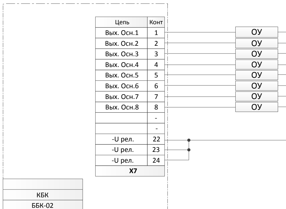
Рисунок 5 – Схема включения основных выходов блока ББК-02
