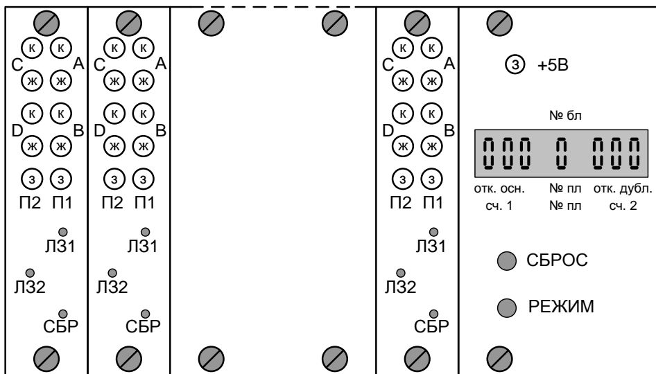
Рисунок 2 – Эскиз передней панели блока приемников К-10
