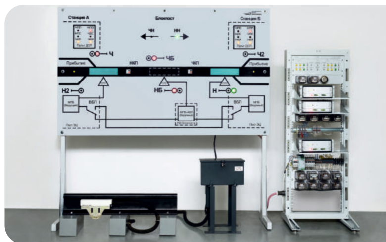
ULIS MPB
